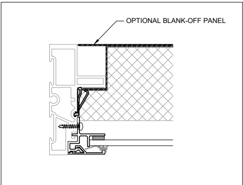
JAMB
