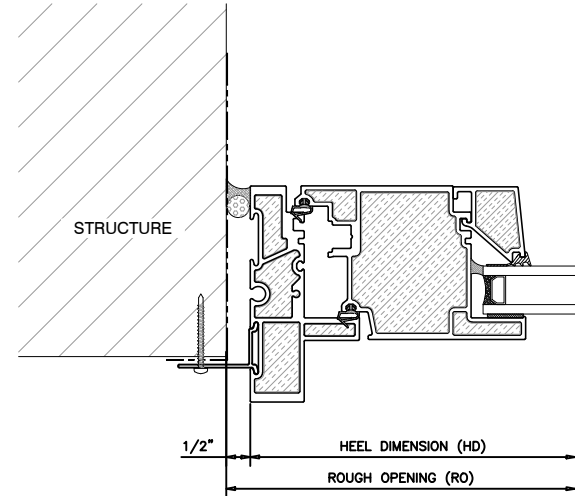
7 INWARD SLIDING DOOR JAMB
