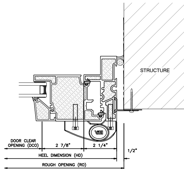
4 OUTSWING DOOR HINGE JAMB
