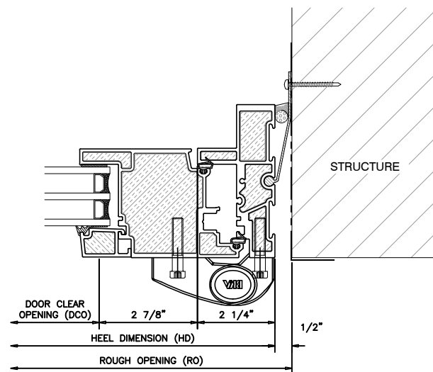
4 OUTSWING DOOR HINGE JAMB OUTSWING UNIVERSAL DOOR
