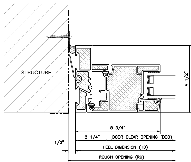
3 OUTSWING DOOR HANDLE JAMB OUTSWING UNIVERSAL DOOR
