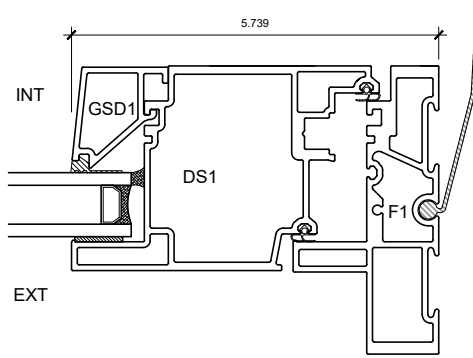
3 OPERABLE JAMB
