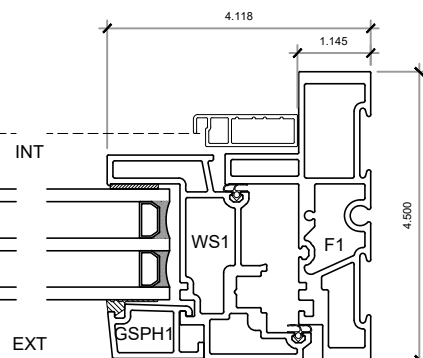
6 OPERABLE JAMB
