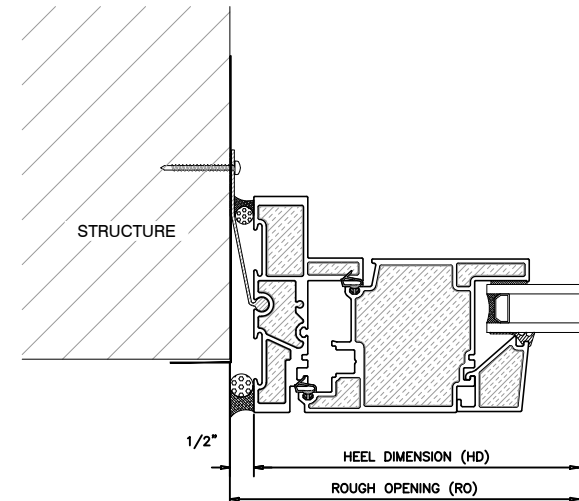
7 SLIDING DOOR JAMB OUTWARD SLIDING DOOR
