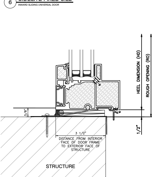
6 SIDELITE FIXED SILL INWARD SLIDING UNIVERSAL DOOR
