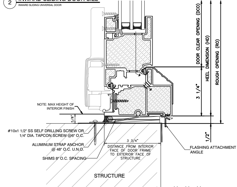
2 INWARD SLIDING DOOR SILL INWARD SLIDING UNIVERSAL DOOR
