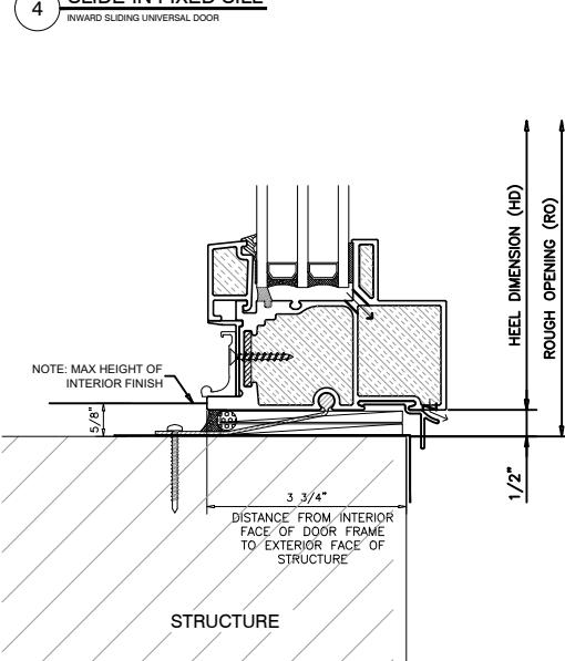
4 SLIDE-IN FIXED SILL INWARD SLIDING UNIVERSAL DOOR
