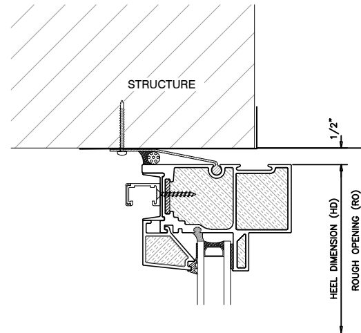
3 SLIDE-IN FIXED HEAD INWARD SLIDING UNIVERSAL DOOR
