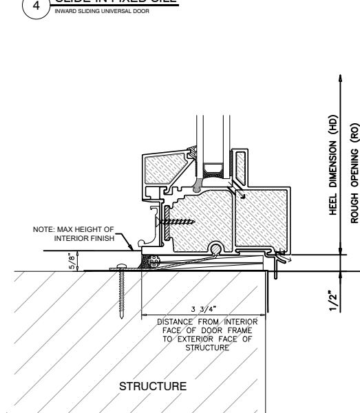
4 SLIDE-IN FIXED SILL INWARD SLIDING UNIVERSAL DOOR
