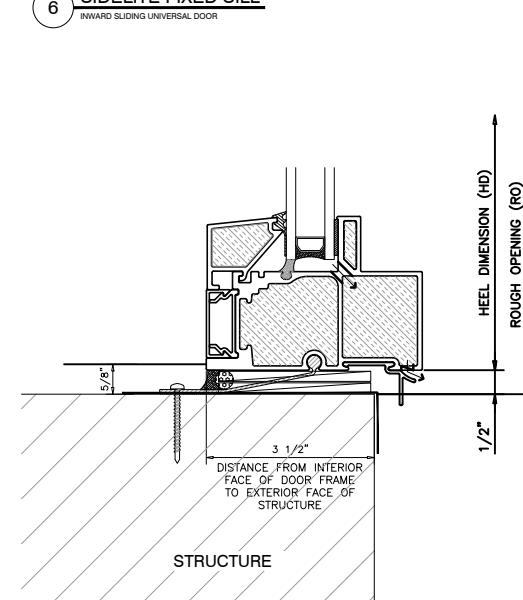
6 SIDELITE FIXED SILL INWARD SLIDING UNIVERSAL DOOR
