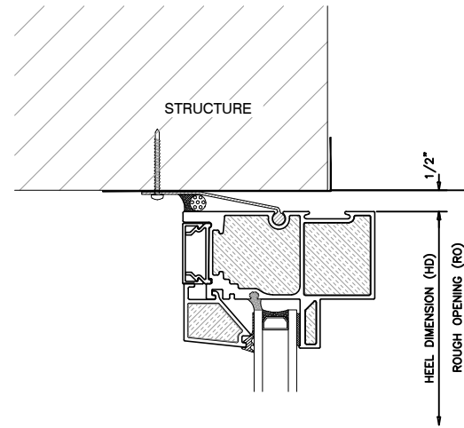
5 SIDELITE FIXED HEAD INWARD SLIDING UNIVERSAL DOOR
