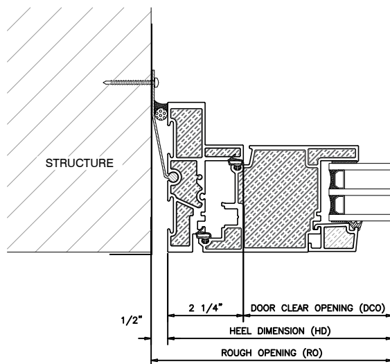
3 OUTSWING DOOR HANDLE JAMB OUTSWING UNIVERSAL DOOR
