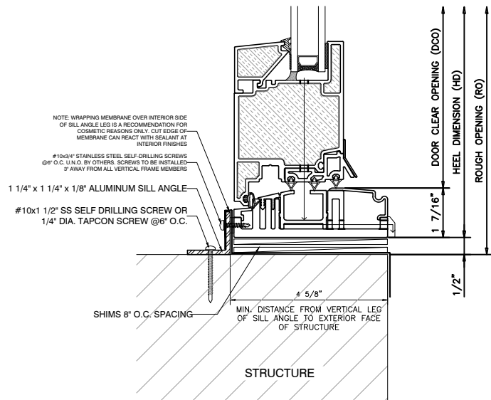
2 INSWING DOOR SILL INSWING UNIVERSAL DOOR
