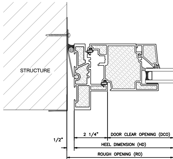
3 INSWING DOOR JAMB - NON HINGED INSWING UNIVERSAL DOOR
