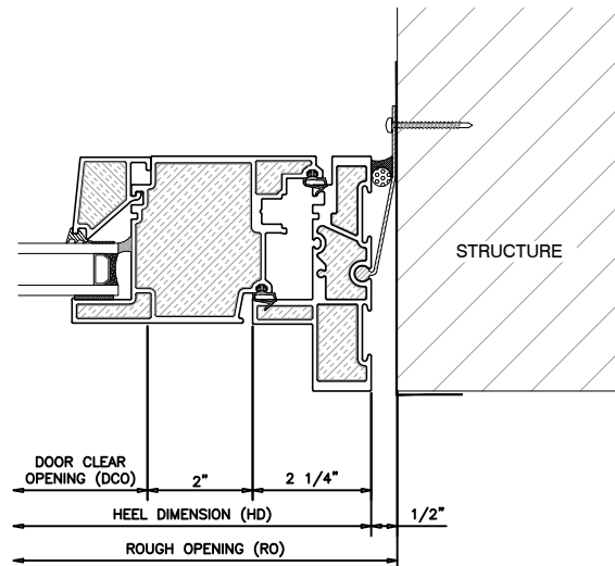
4 INSWING DOOR JAMB - HINGED INSWING UNIVERSAL DOOR
