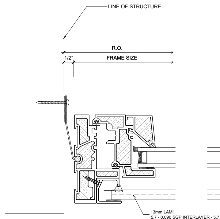
A OPERABLE JAMB H1 SCALE: 4"=1'-0"
