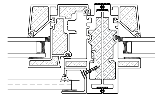
B COUPLER H1 SCALE: 4"=1'-0"
