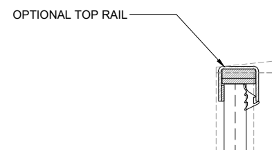
E GUARDRAIL SECTION H1 SCALE: 4"=1'-0"
