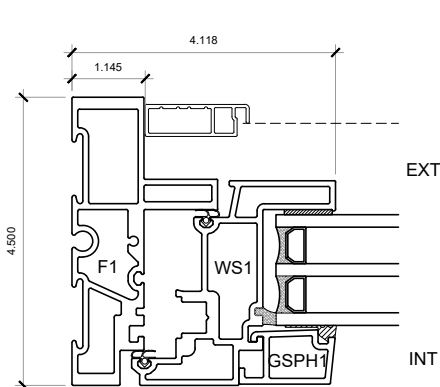
6 OPERABLE JAMB
