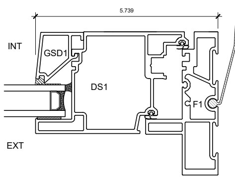
3 OPERABLE JAMB
