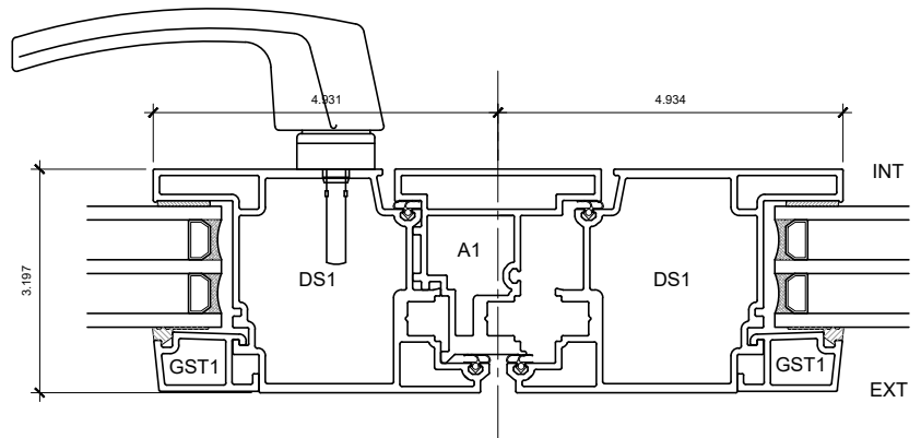
6 ASTRAGAL
