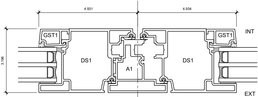
6 ASTRAGAL
