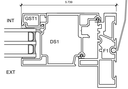
3 OPERABLE JAMB
